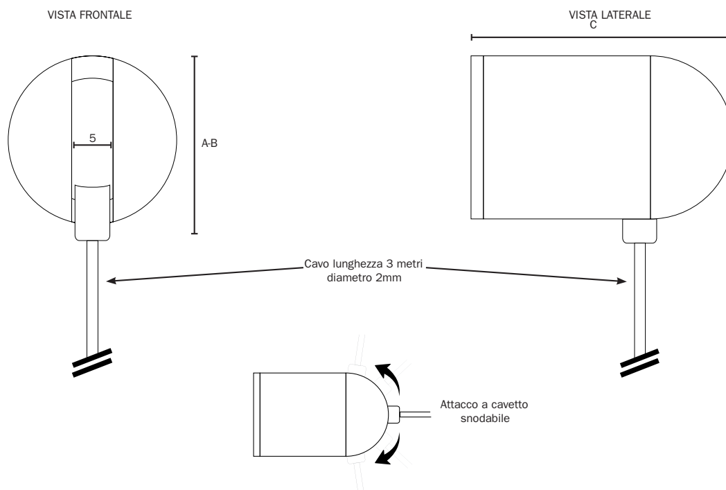
DIMENSIONI PRODOTTO (mm)
